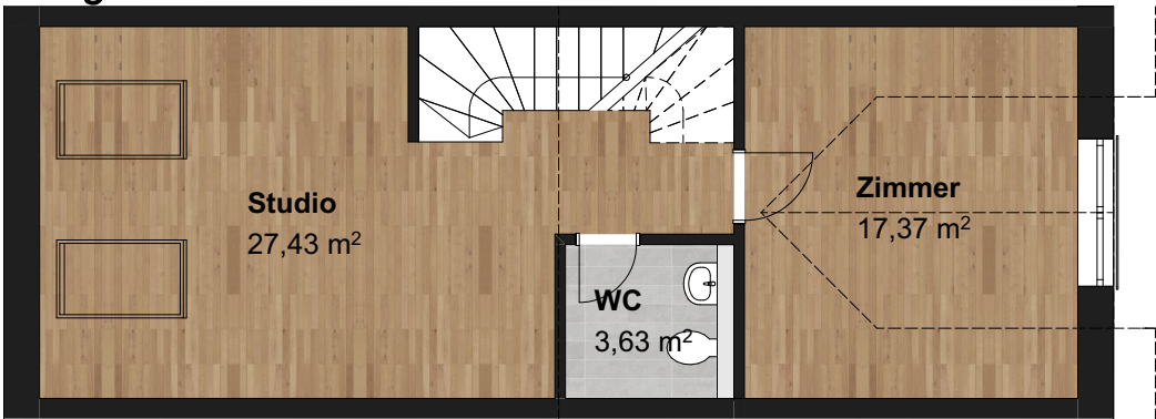
Grundriss Dachgeschoss
