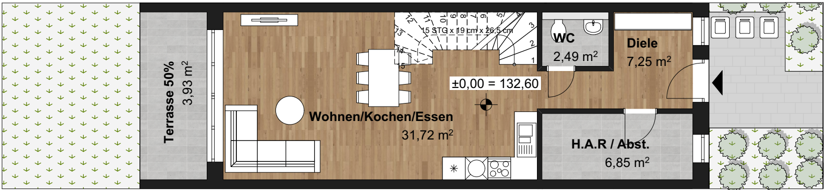
Grundriss Erdgeschoss
