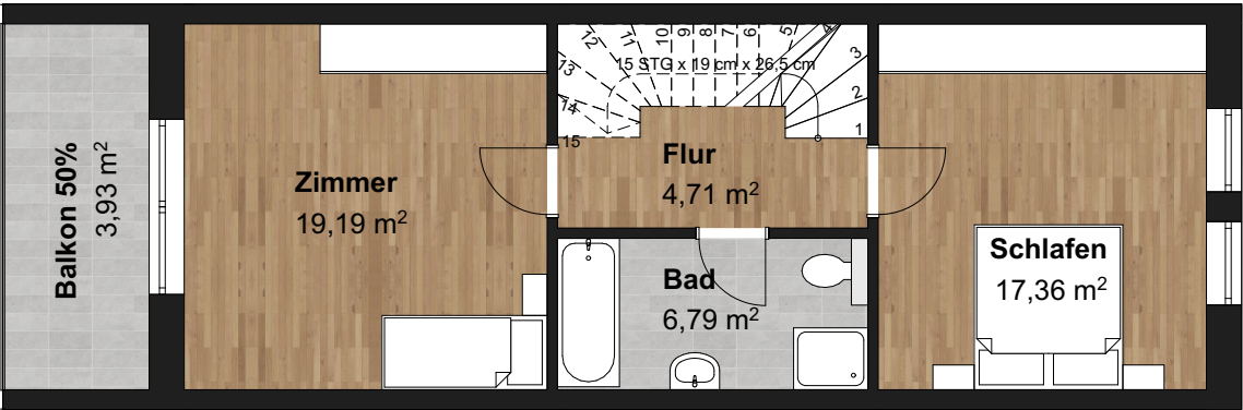
Grundriss Obergeschoss
