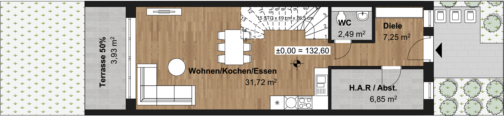
Grundriss Erdgeschoss
